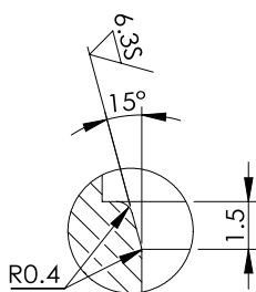
細部放大圖 A
