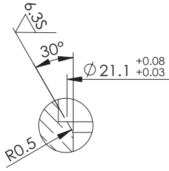
細部放大圖 B
