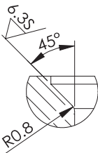
細部放大圖 A
