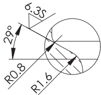
細部放大圖 B
