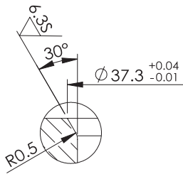
細部放大圖 B
