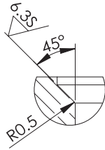
細部放大圖 A
