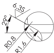
細部放大圖 B
