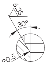
細部放大圖 B
